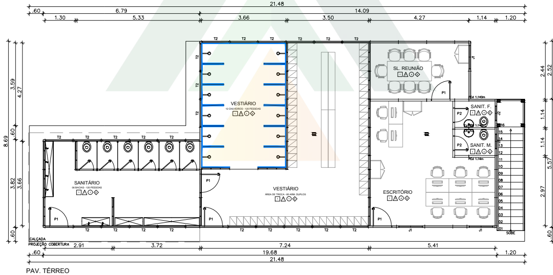
PAV. TÉRREO
