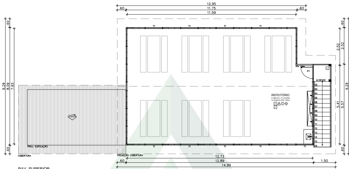
PAV. SUPERIOR
